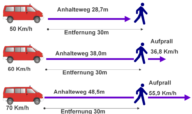
Erläuterung zur Grafik: Bei der Darstellung handelt es sich um den Anhalteweg bei einer Gefahrenbremsung.
